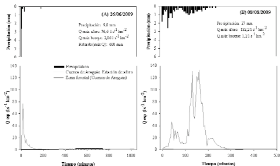
Figura 6. Hidrogramas y hietogramas para 2 eventos registrados en la cuenca de Araguás en condiciones secas. Nótese que la escala en el eje de ordenadas varía en cada caso.
