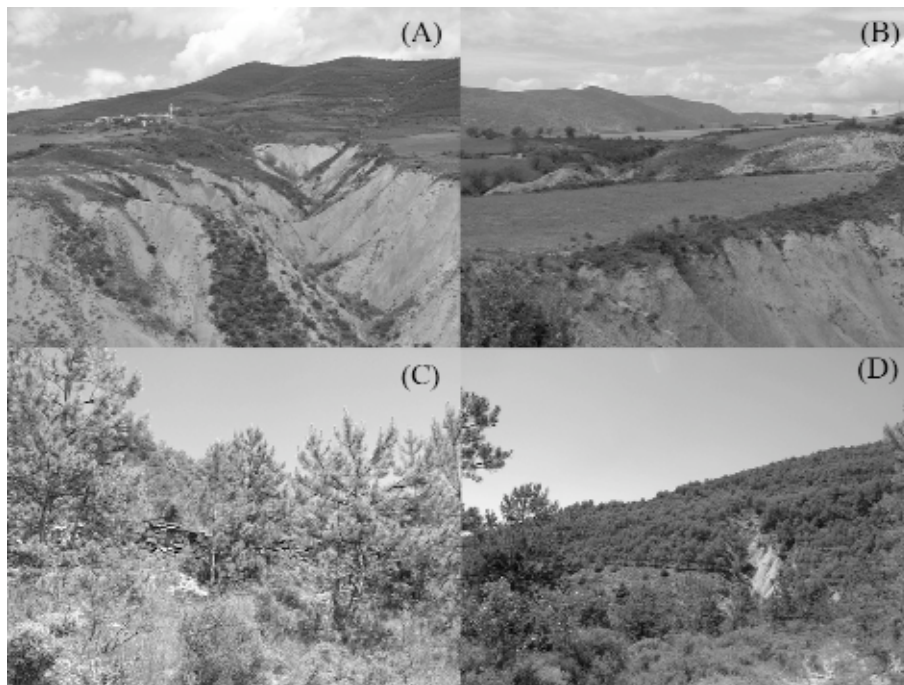
Figura 2. Cuenca de Araguás. A. Desarrollo de cárcavas en la parte baja de la cuenca. B. Prados, matorrales y campos abandonados en la parte media de la cuenca. C. Recolonización vegetal en antiguas terrazas de cultivo. D. Área forestal en la parte superior de la cuenca.
