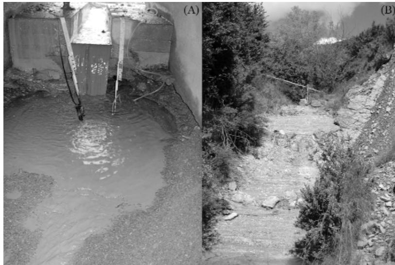
Figura 3. A. Estación de aforo y canal de estiaje en la cuenca de Araguás. B. Sonda de nivel instalada a la salida de la zona forestal de la cuenca de Araguás.
